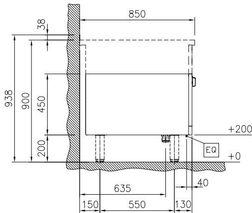
Zij aanzicht
